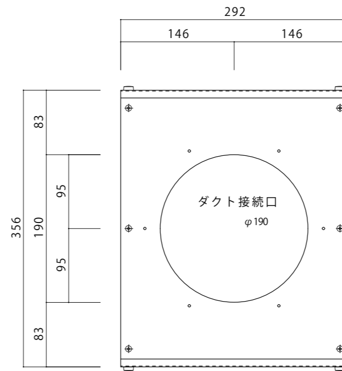
上面/底面
